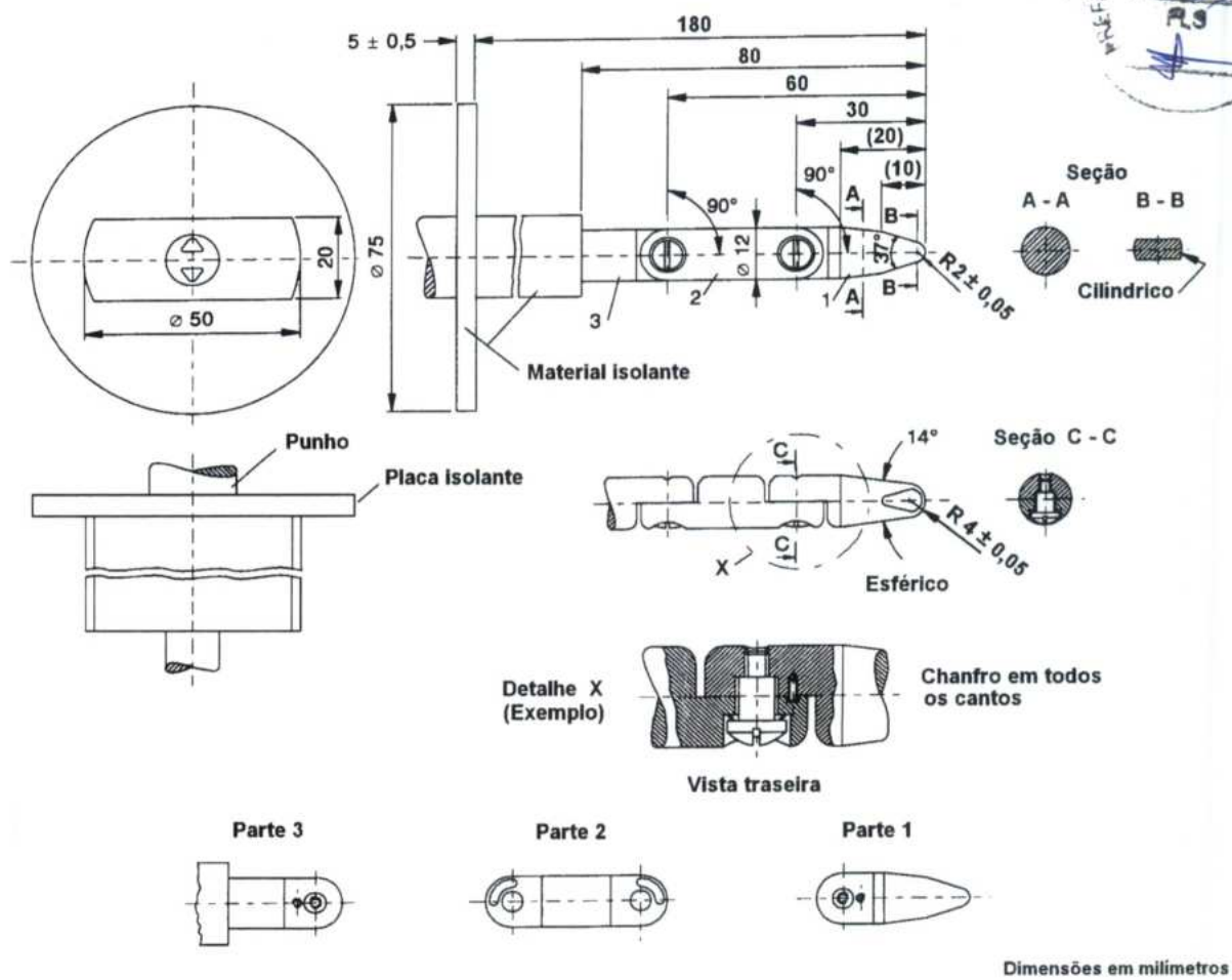
Figura 8-a) – Dedo-de-prova
