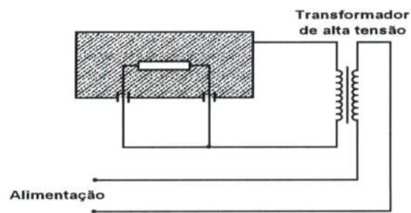
Figura 11-b) - Esquema para ensaio de isolamento elétrico
