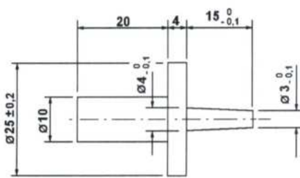
Figura 8-b) – Pino-de-prova
