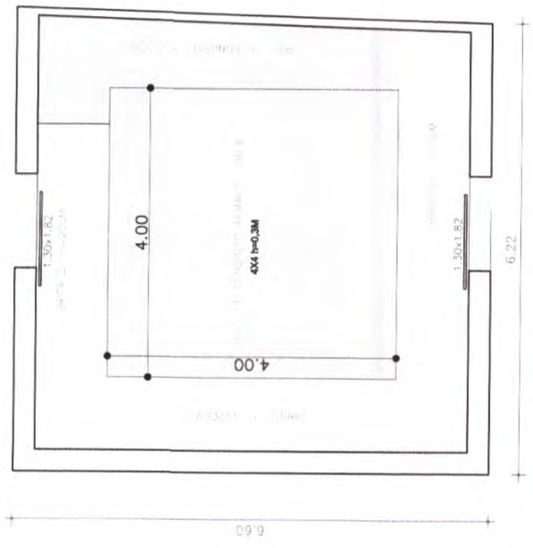
PLANTA BAIXA BASE esc 1:30
